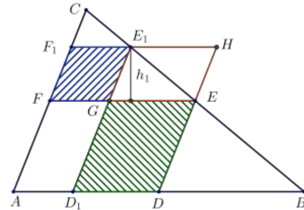
Joon. 8. Suurima pindalaga rööpküliku ülesande Eukleidese lahendust abistav joonis.
