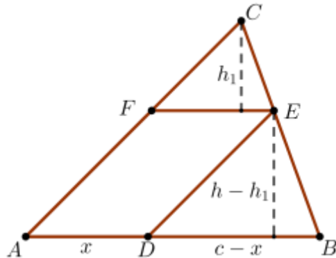
Joon. 7. Suurima pindalaga rööpküliku ülesande tuletisega lahendust selgitav joonis.
