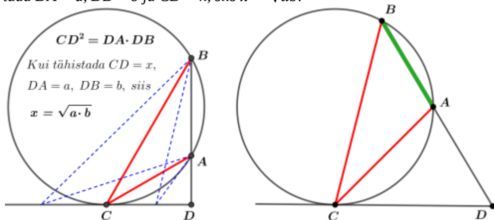
Joon. 5. Eukleidese lahendus ja selle rakendamisvõimalus kaldekraanide puhul.
