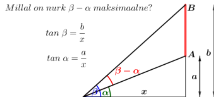
Joon. 4. Suurima vaatenurga ülesande lähtejoonis.
