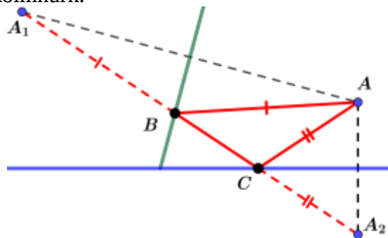
Joon. 3. Vähima ümbermõõduga kolmnurga ülesande lahenduse joonis.
