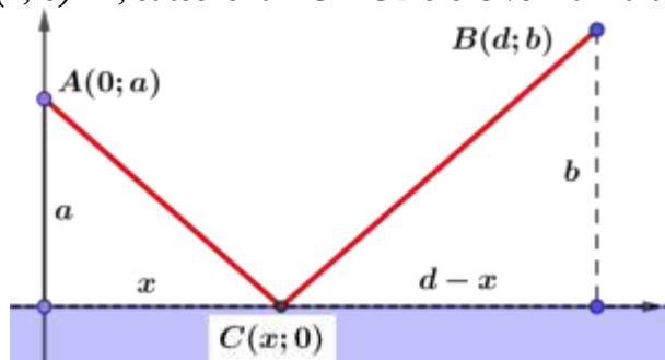
Joon. 1. Lühima teekonna ülesande joonis tuletisega lahenduskäigu puhul.
