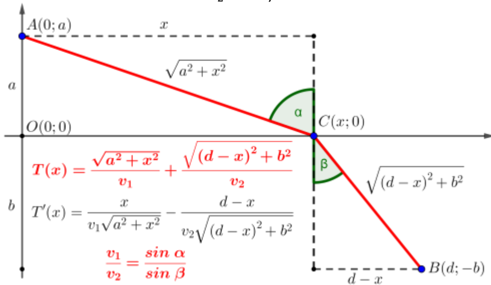
Joon. 6. Snelliuse valguse murdumisseaduse tuletuskäiku selgitav joonis.
