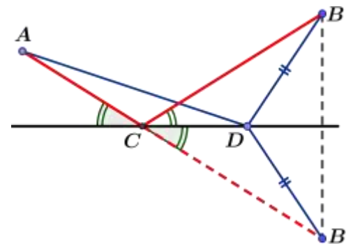
Joon. 2. Lühima teekonna ülesande Heroni lahenduskäigu joonis.
